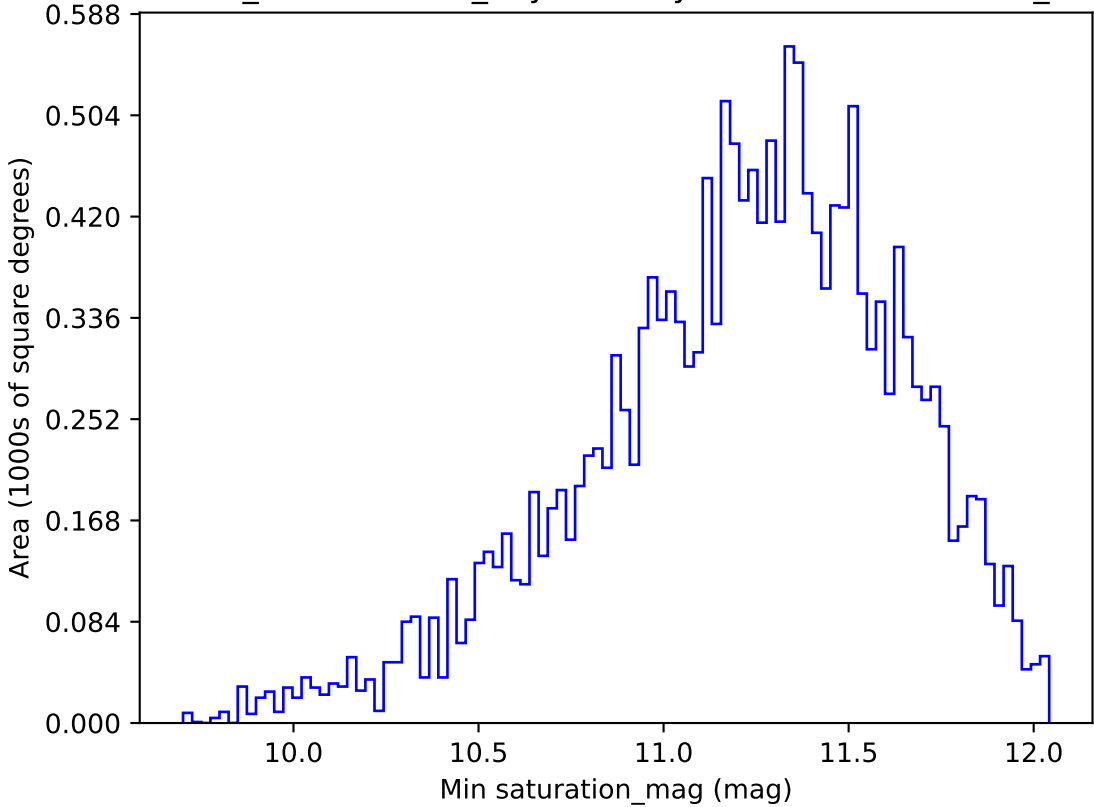
weather_cloudso2v3.4_10yrs WFD y band: Min saturation_mag
