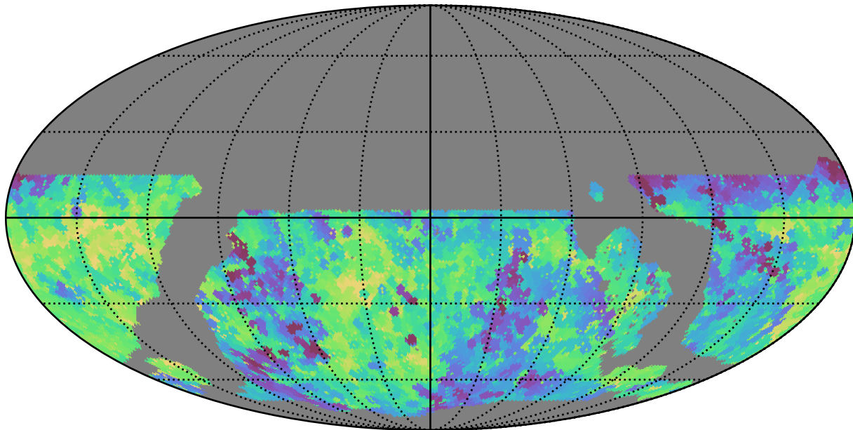
weather_cloudso2v3.4_10yrs WFD u band: Min saturation_mag
