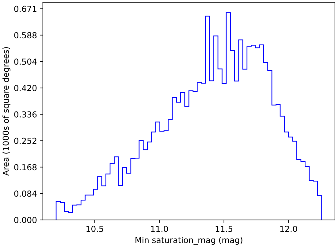
weather_cloudso2v3.4_10yrs WFD u band: Min saturation_mag
