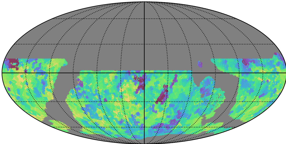
weather_cloudso2v3.4_10yrs WFD r band: Min saturation_mag
