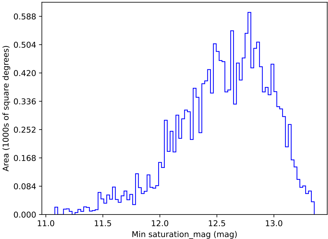
weather_cloudso2v3.4_10yrs WFD r band: Min saturation_mag
