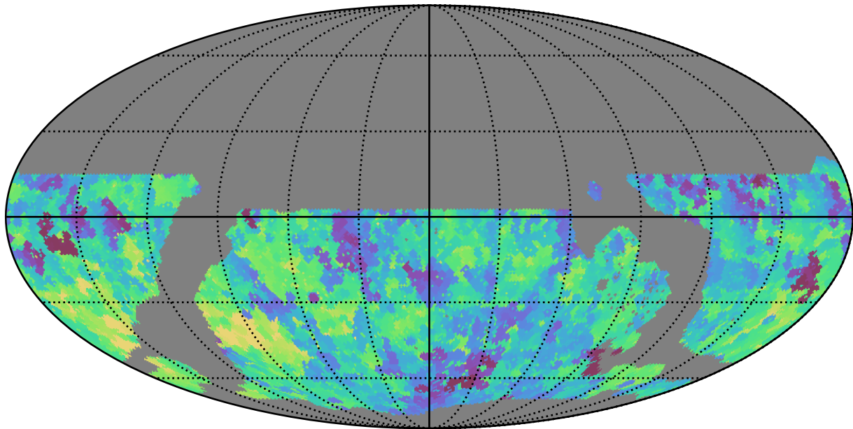
weather_cloudso2v3.4_10yrs WFD i band: Min saturation_mag
