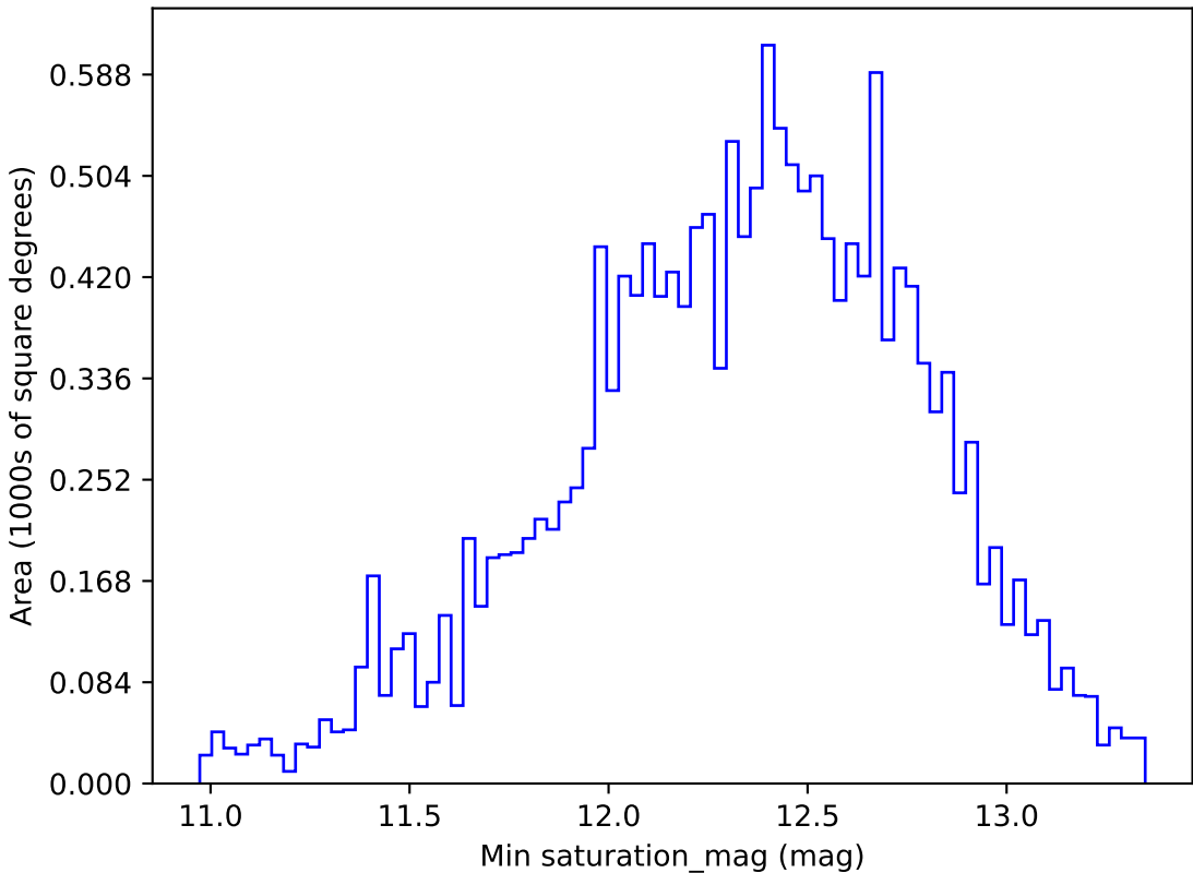
weather_cloudso2v3.4_10yrs WFD i band: Min saturation_mag
