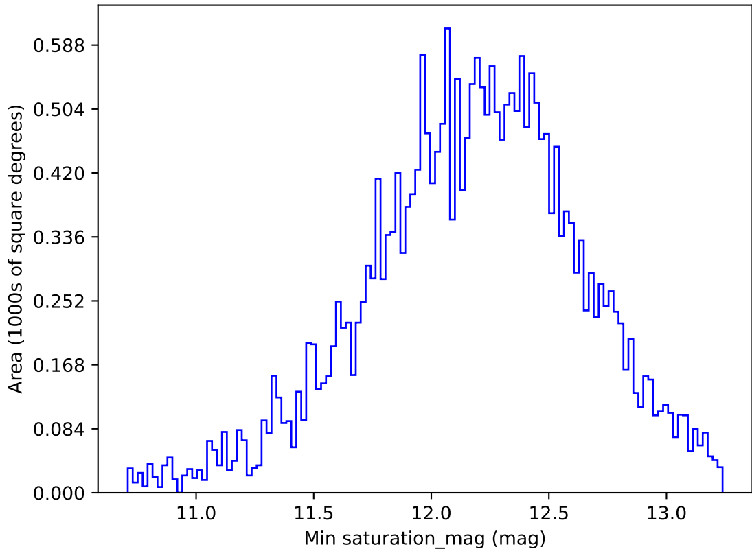
weather_cloudso2v3.4_10yrs All sky z band: Min saturation_mag
