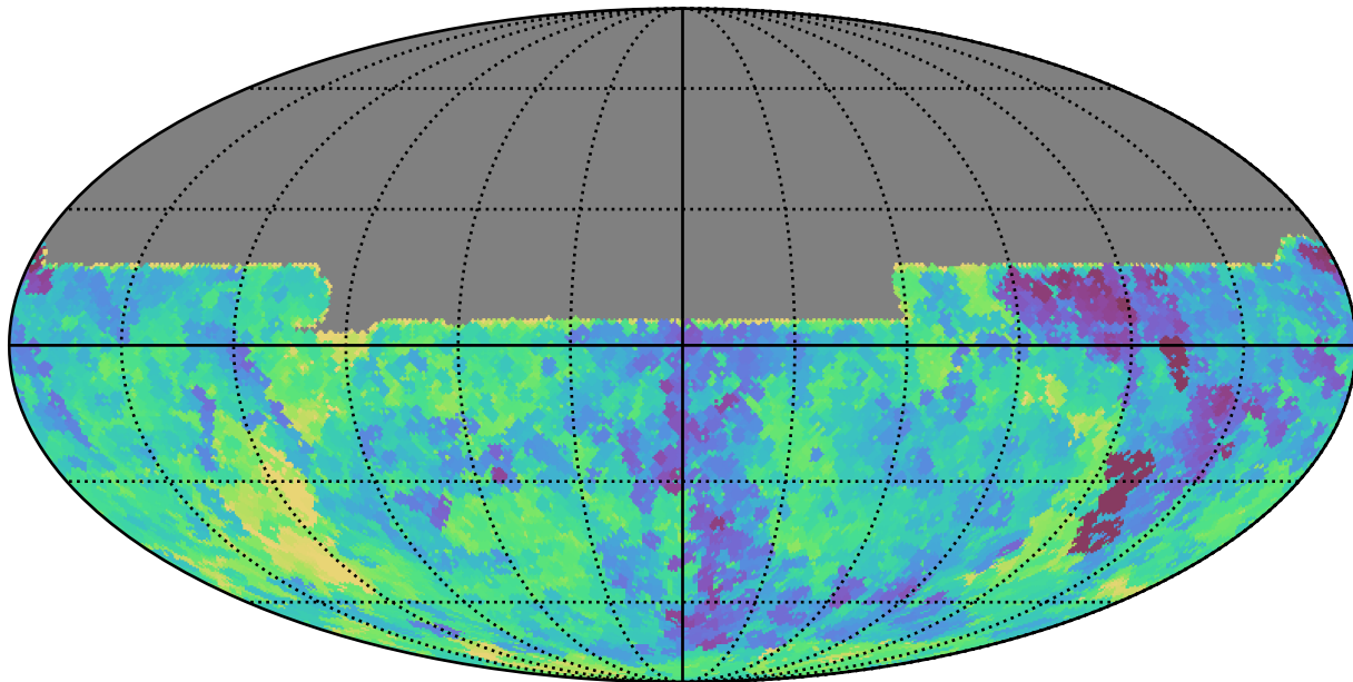
weather_cloudso2v3.4_10yrs All sky y band: Min saturation_mag
