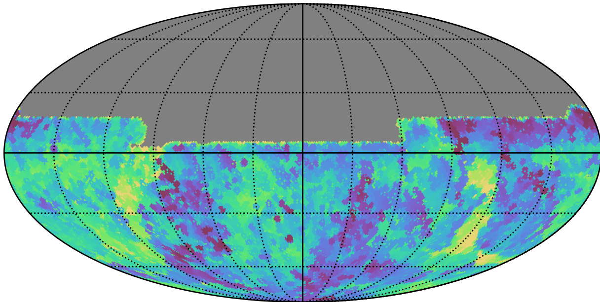
weather_cloudso2v3.4_10yrs All sky u band: Min saturation_mag
