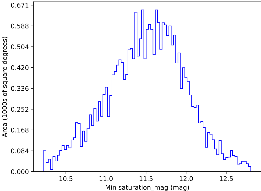
weather_cloudso2v3.4_10yrs All sky u band: Min saturation_mag
