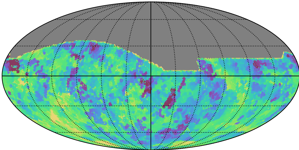
weather_cloudso2v3.4_10yrs All sky r band: Min saturation_mag
