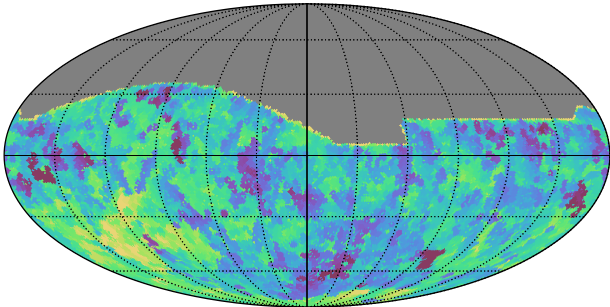
weather_cloudso2v3.4_10yrs All sky i band: Min saturation_mag
