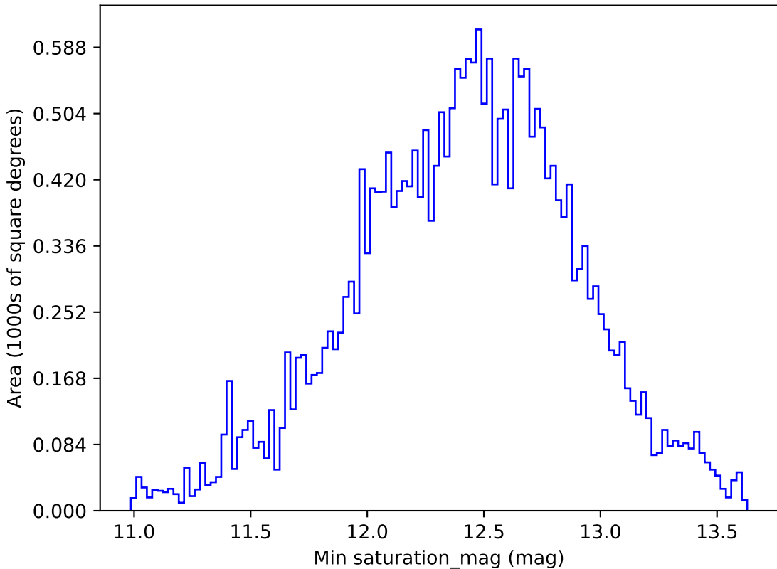
weather_cloudso2v3.4_10yrs All sky i band: Min saturation_mag
