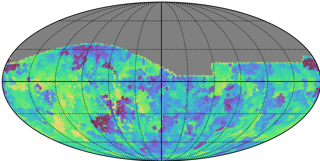
weather_cloudso2v3.4_10yrs All sky g band: Min saturation_mag
