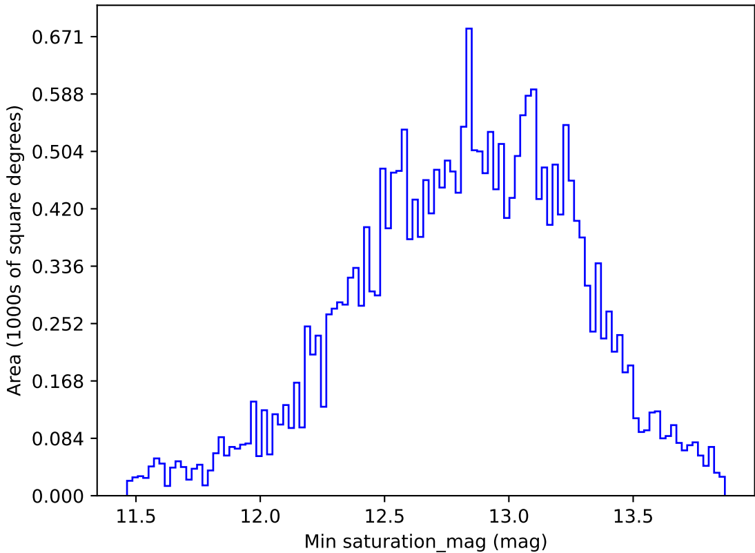
weather_cloudso2v3.4_10yrs All sky g band: Min saturation_mag
