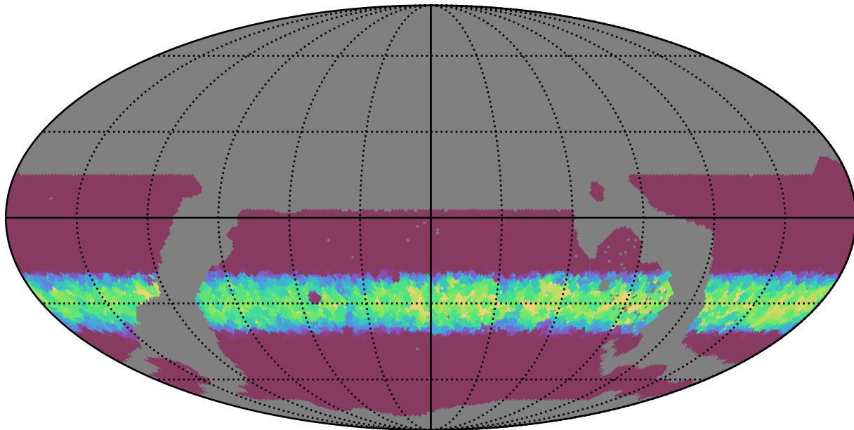
weather_cloudso2v3.4_10yrs WFD z band: Min normairmass
