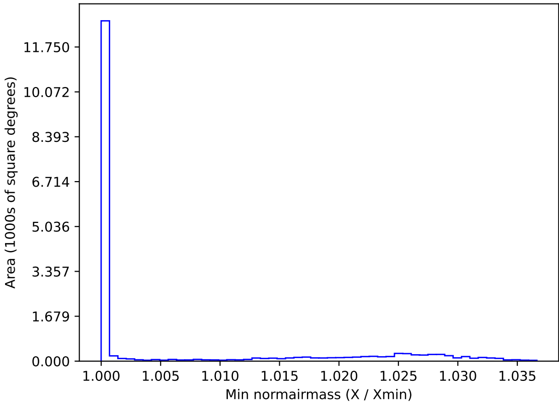
weather_cloudso2v3.4_10yrs WFD z band: Min normairmass
