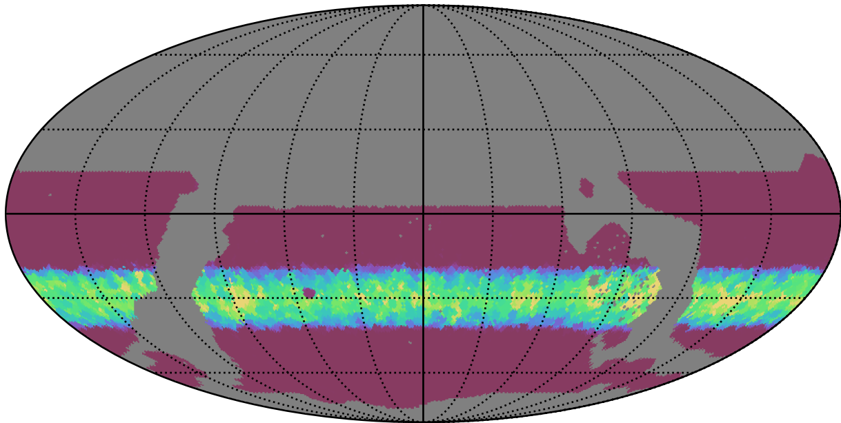
weather_cloudso2v3.4_10yrs WFD y band: Min normairmass
