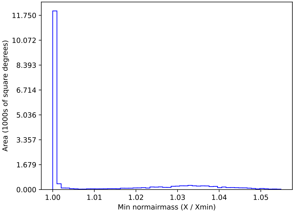
weather_cloudso2v3.4_10yrs WFD u band: Min normairmass
