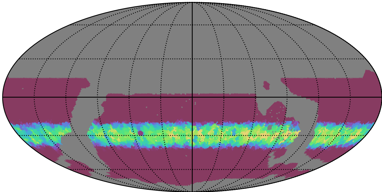
weather_cloudso2v3.4_10yrs WFD r band: Min normairmass
