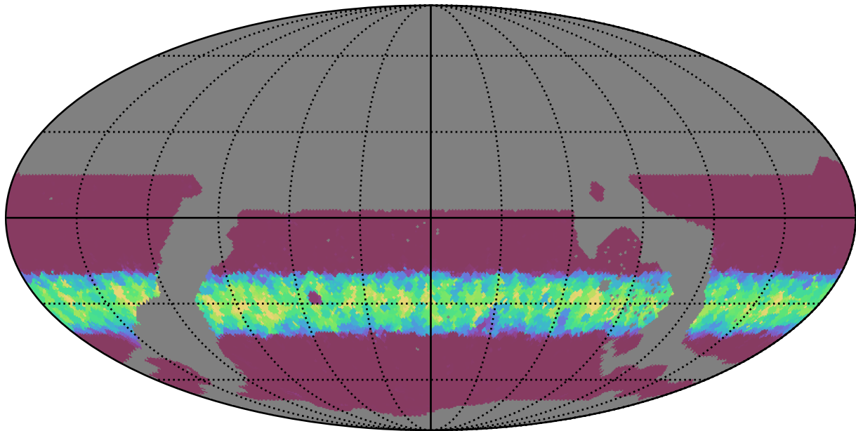
weather_cloudso2v3.4_10yrs WFD g band: Min normairmass
