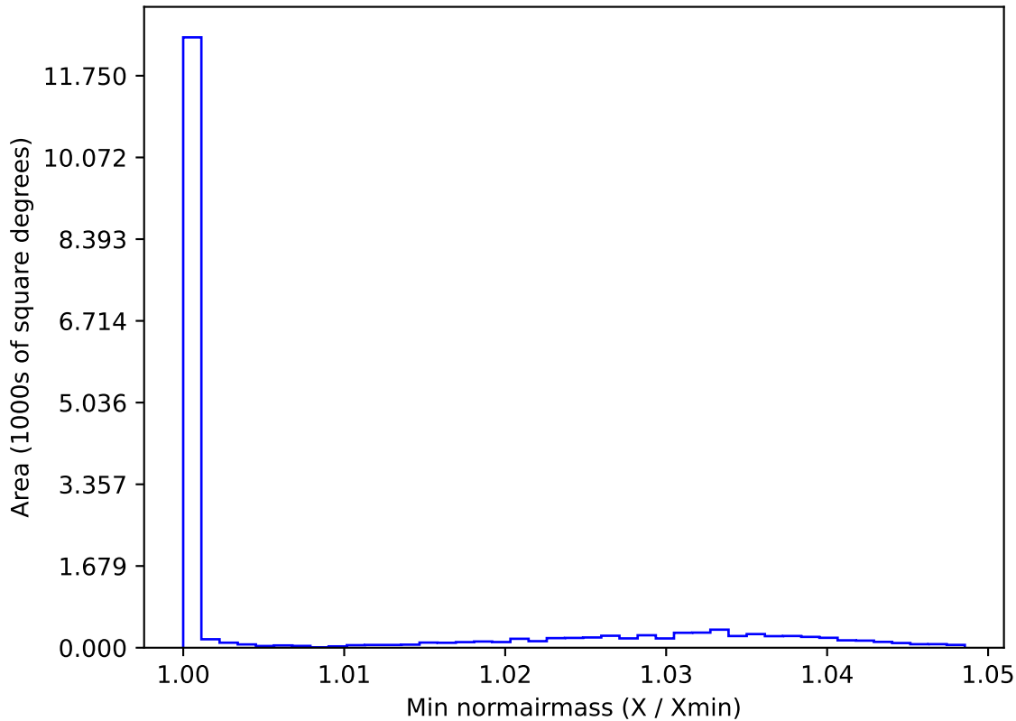
weather_cloudso2v3.4_10yrs WFD g band: Min normairmass
