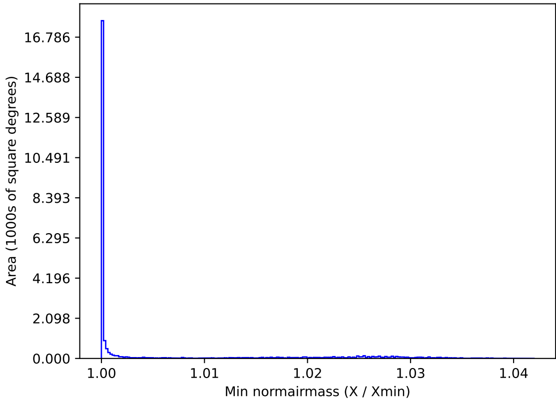
weather_cloudso2v3.4_10yrs All sky z band: Min normairmass
