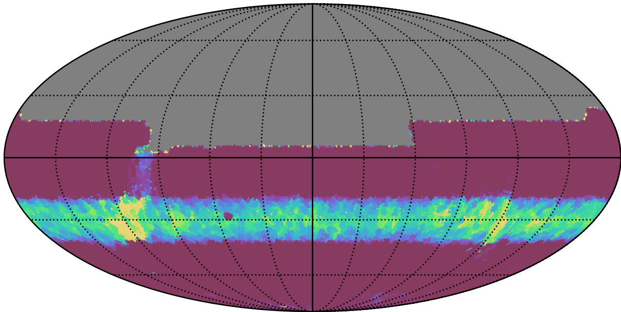
weather_cloudso2v3.4_10yrs All sky y band: Min normairmass
