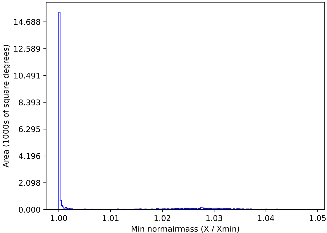
weather_cloudso2v3.4_10yrs All sky y band: Min normairmass
