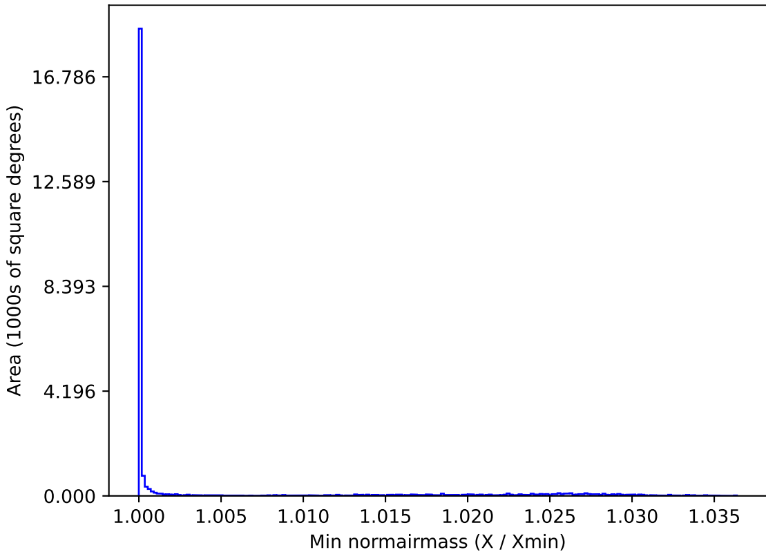
weather_cloudso2v3.4_10yrs All sky i band: Min normairmass
