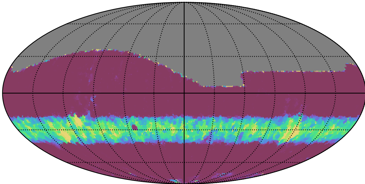
weather_cloudso2v3.4_10yrs All sky g band: Min normairmass
