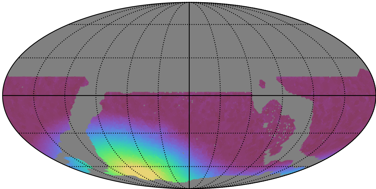
weather_cloudso2v3.4_10yrs WFD z band: Min moonDistance
