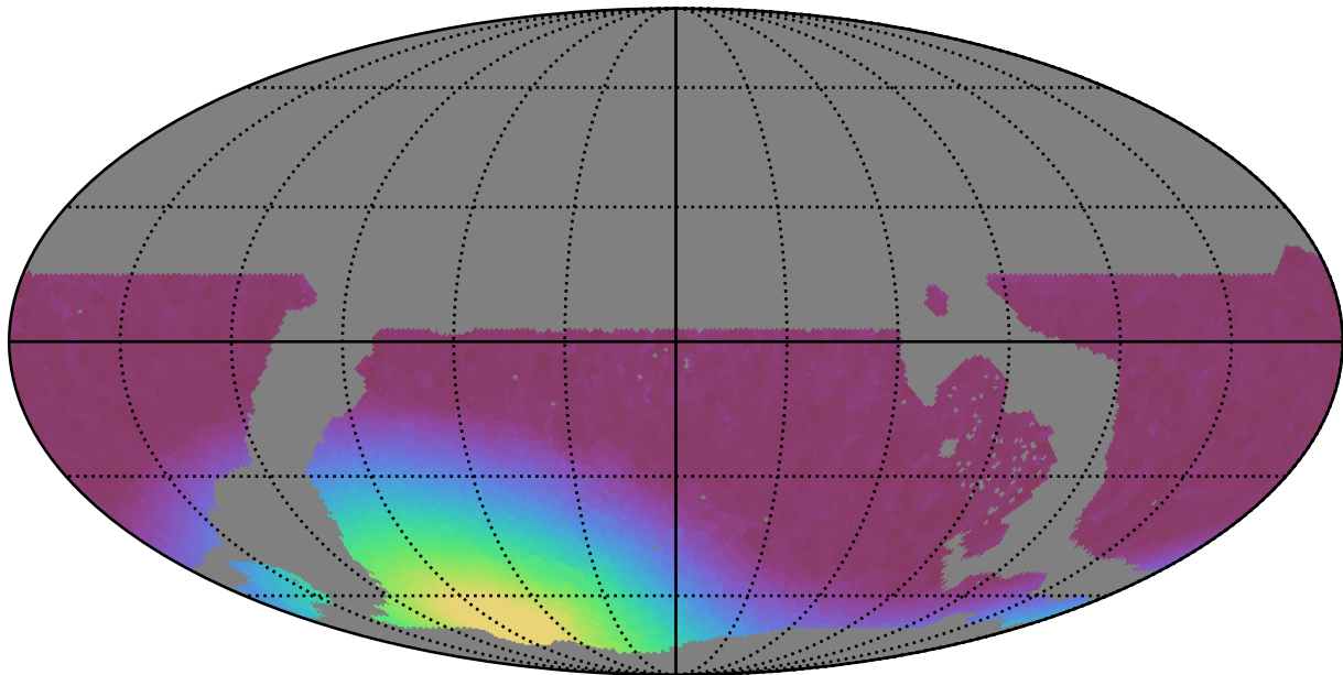
weather_cloudso2v3.4_10yrs WFD y band: Min moonDistance
