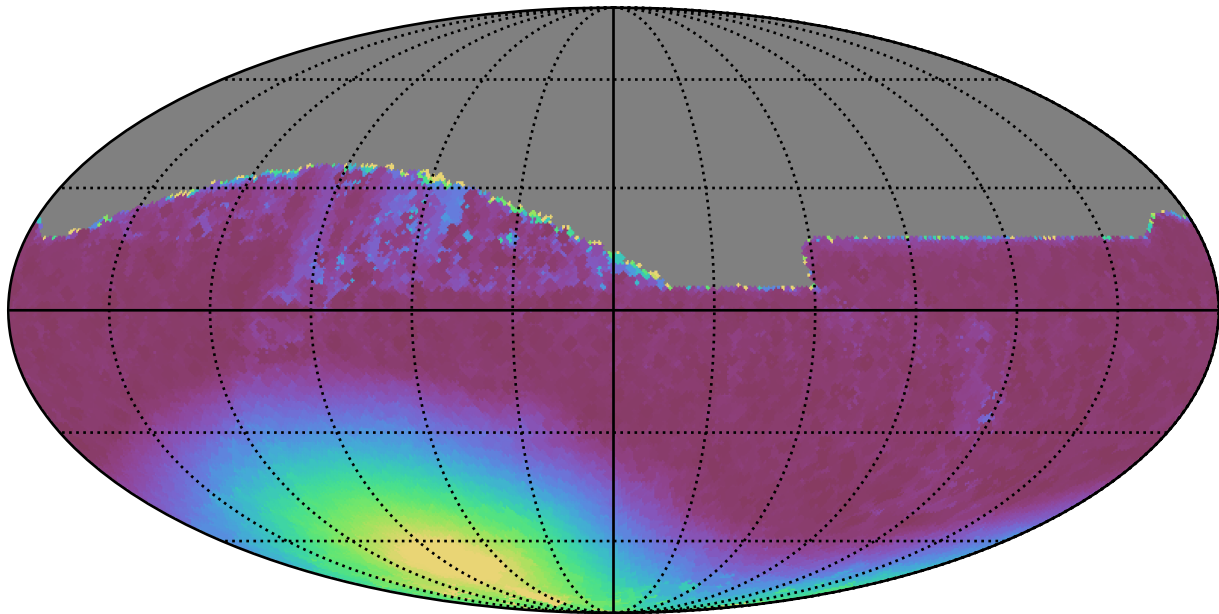
weather_cloudso2v3.4_10yrs All sky z band: Min moonDistance
