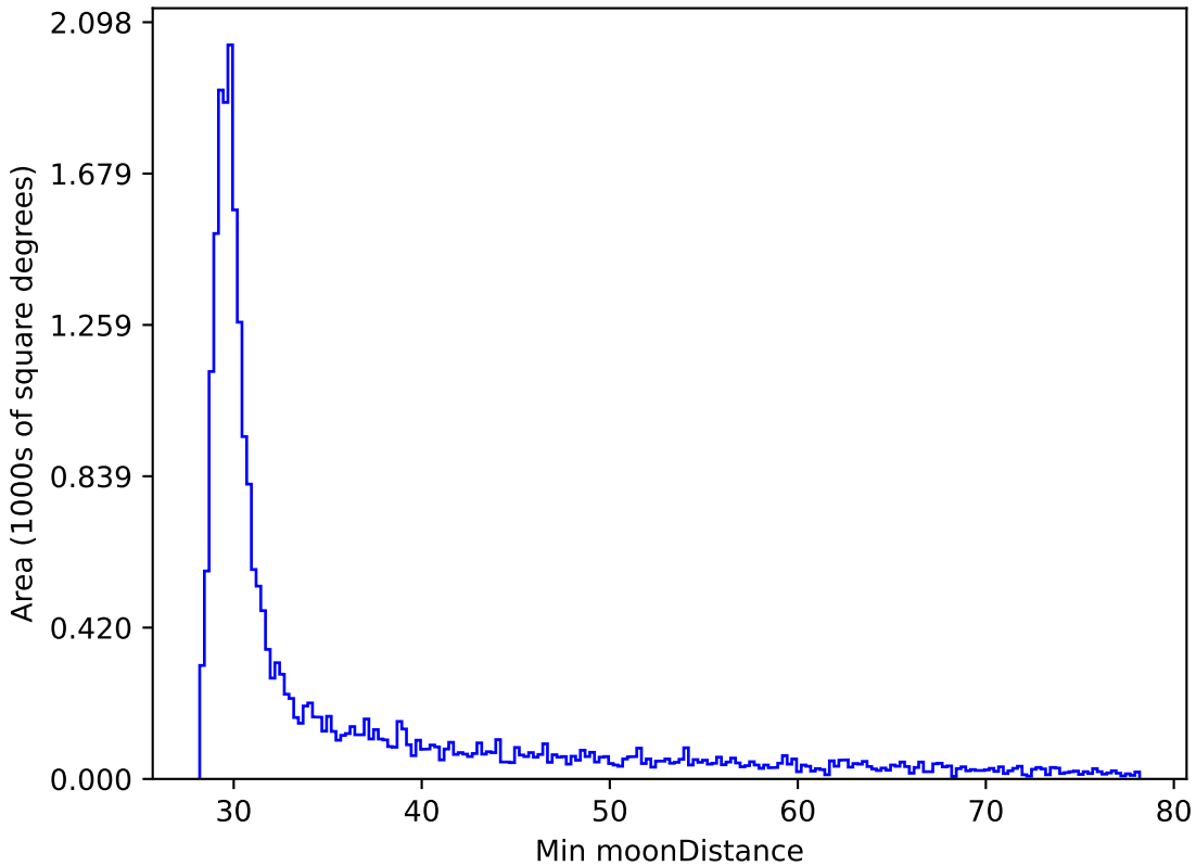
weather_cloudso2v3.4_10yrs All sky z band: Min moonDistance
