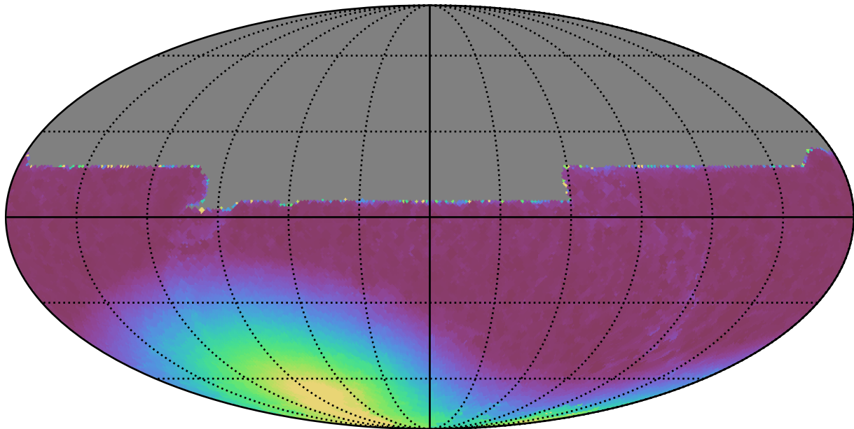
weather_cloudso2v3.4_10yrs All sky y band: Min moonDistance
