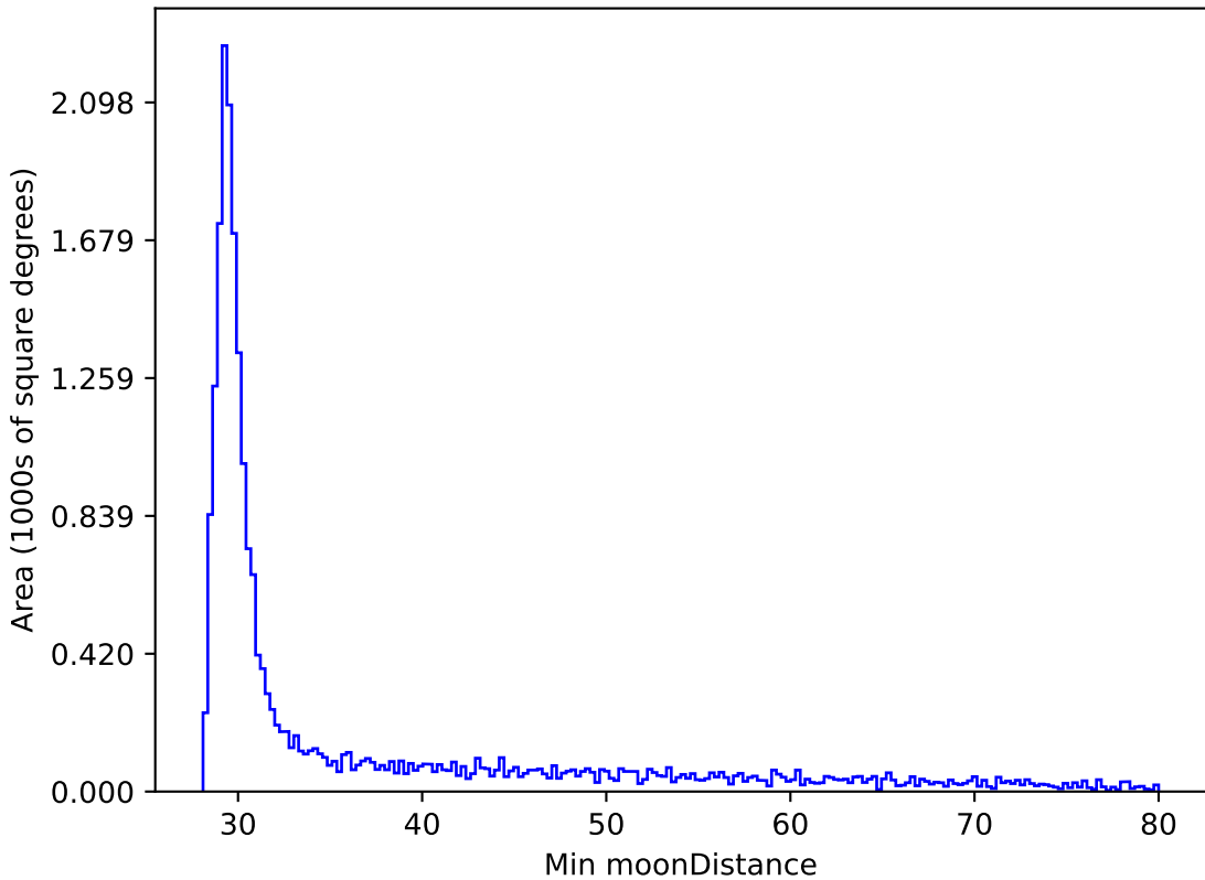
weather_cloudso2v3.4_10yrs All sky y band: Min moonDistance
