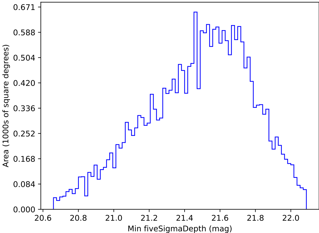
weather_cloudso2v3.4_10yrs Yr 1 y band: Min fiveSigmaDepth
