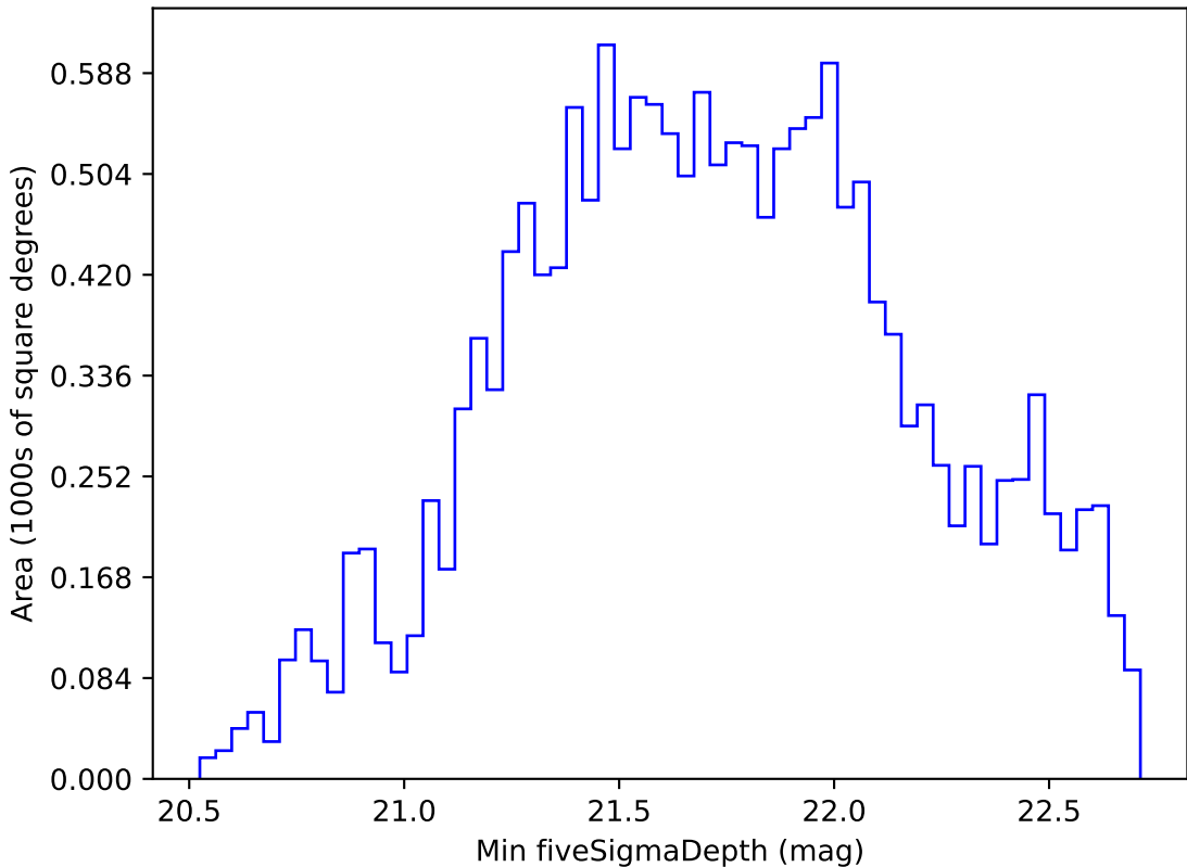
weather_cloudso2v3.4_10yrs WFD i band: Min fiveSigmaDepth
