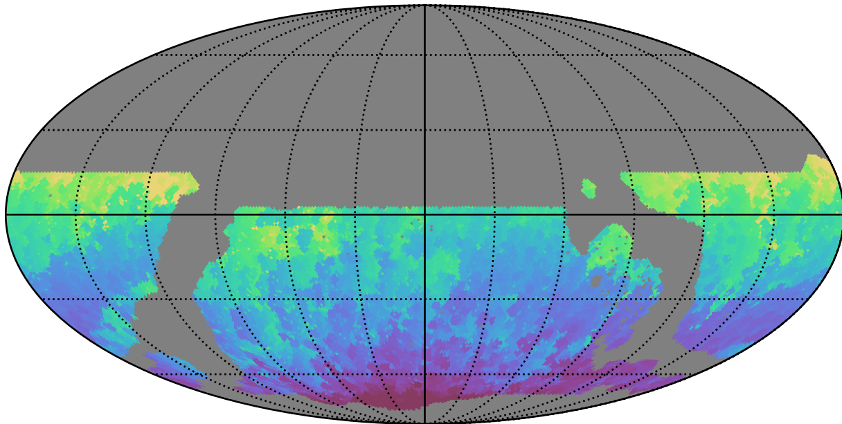
weather_cloudso2v3.4_10yrs WFD z band: Min HA
