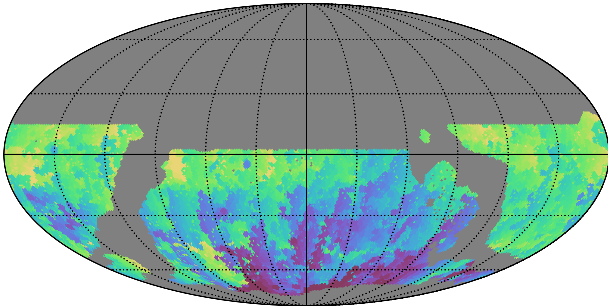
weather_cloudso2v3.4_10yrs WFD u band: Min HA
