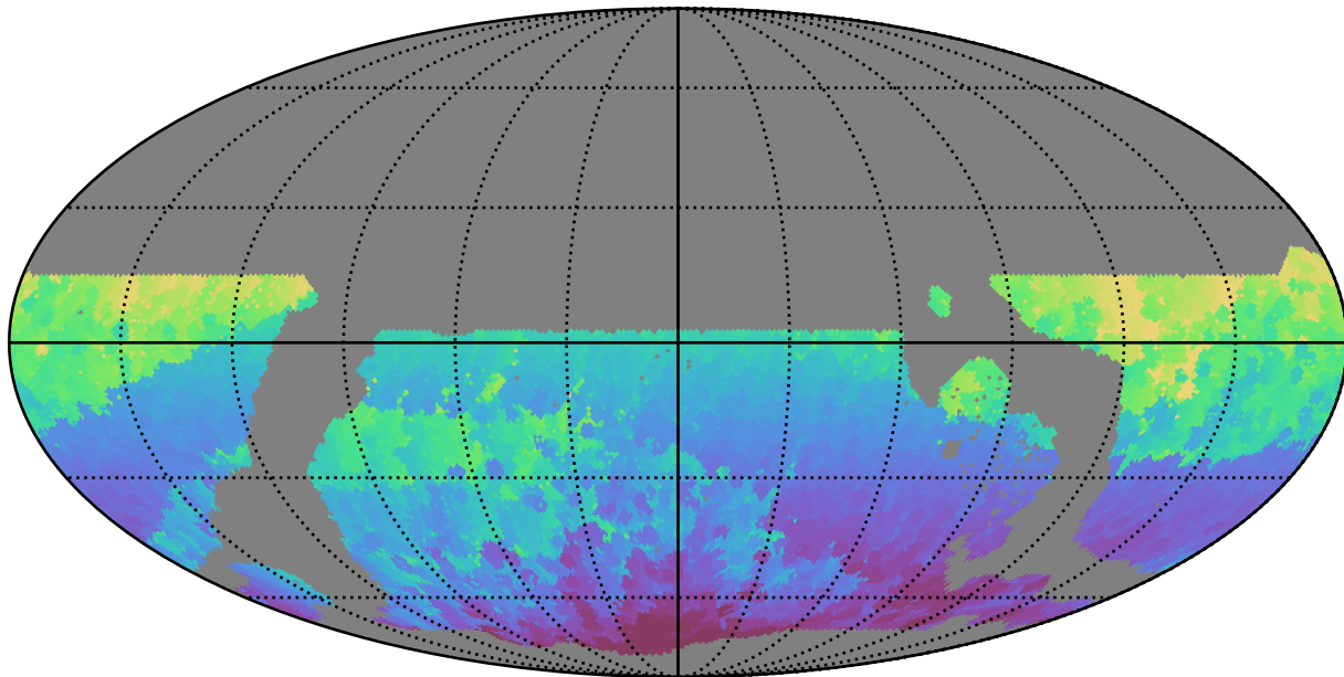
weather_cloudso2v3.4_10yrs WFD r band: Min HA
