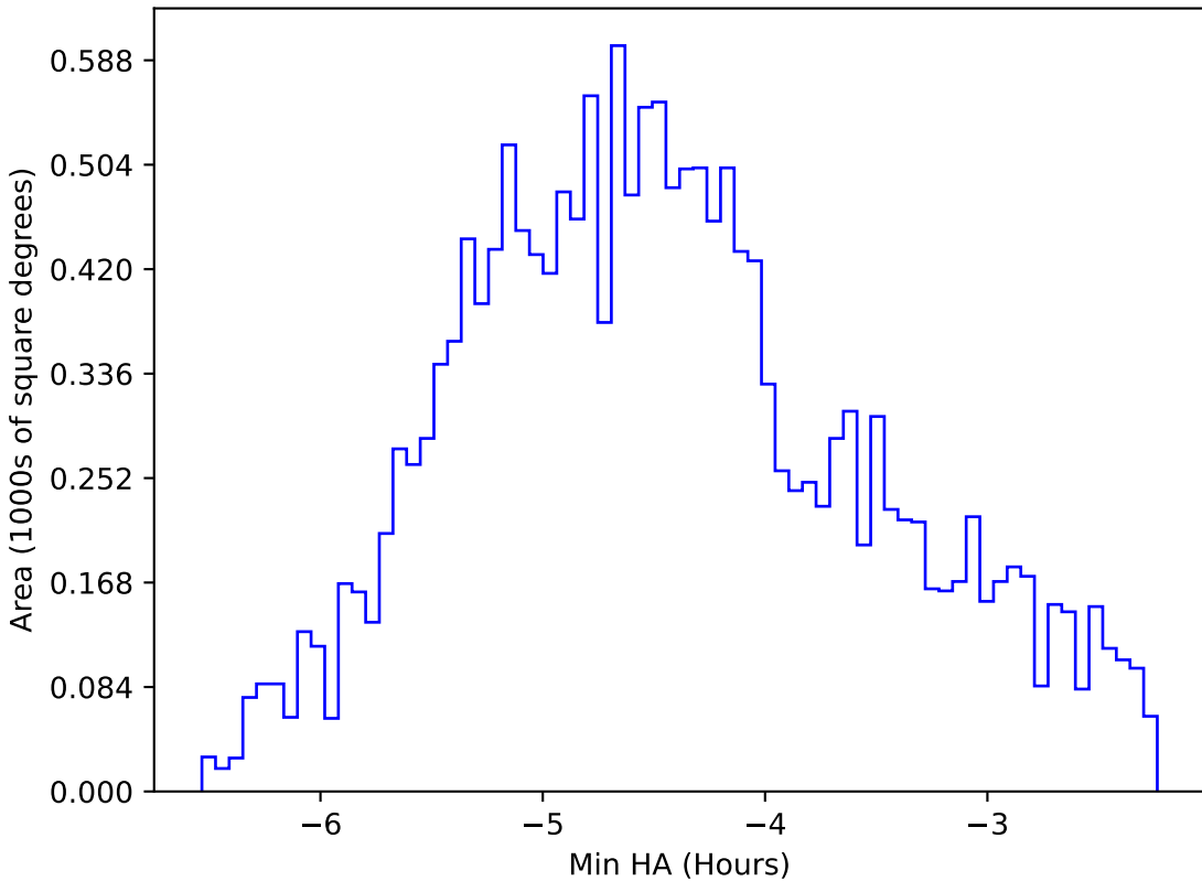
weather_cloudso2v3.4_10yrs WFD r band: Min HA
