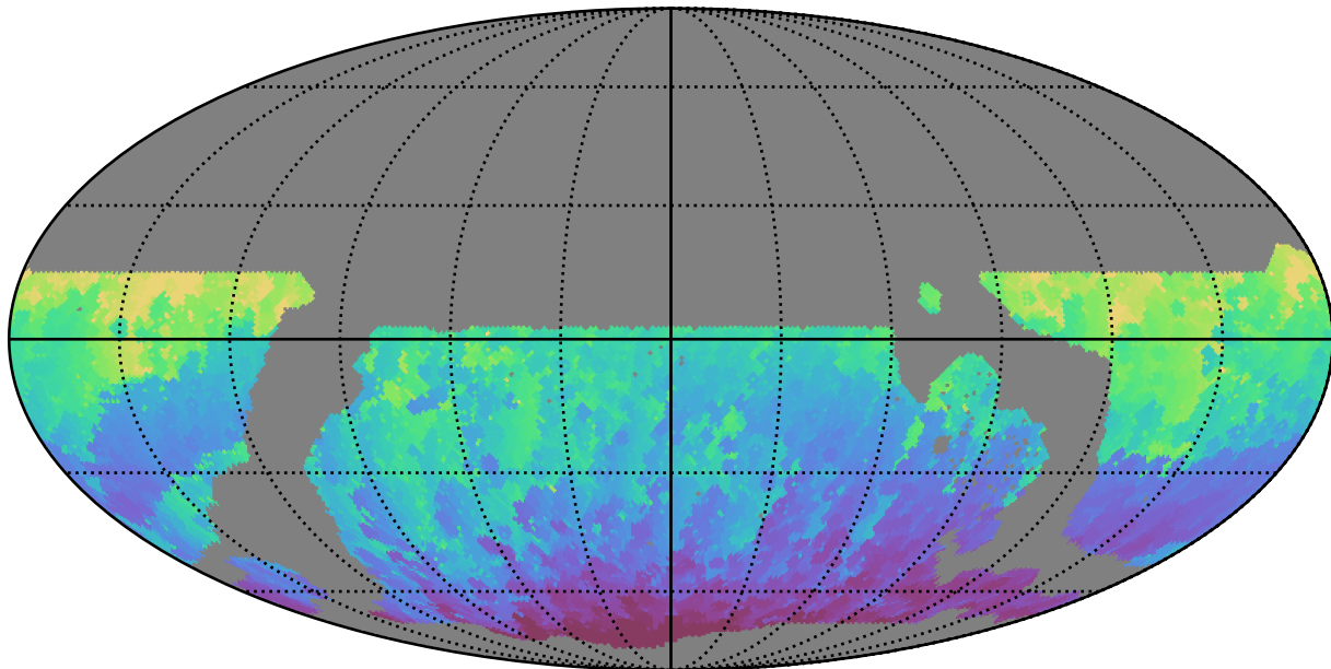
weather_cloudso2v3.4_10yrs WFD i band: Min HA
