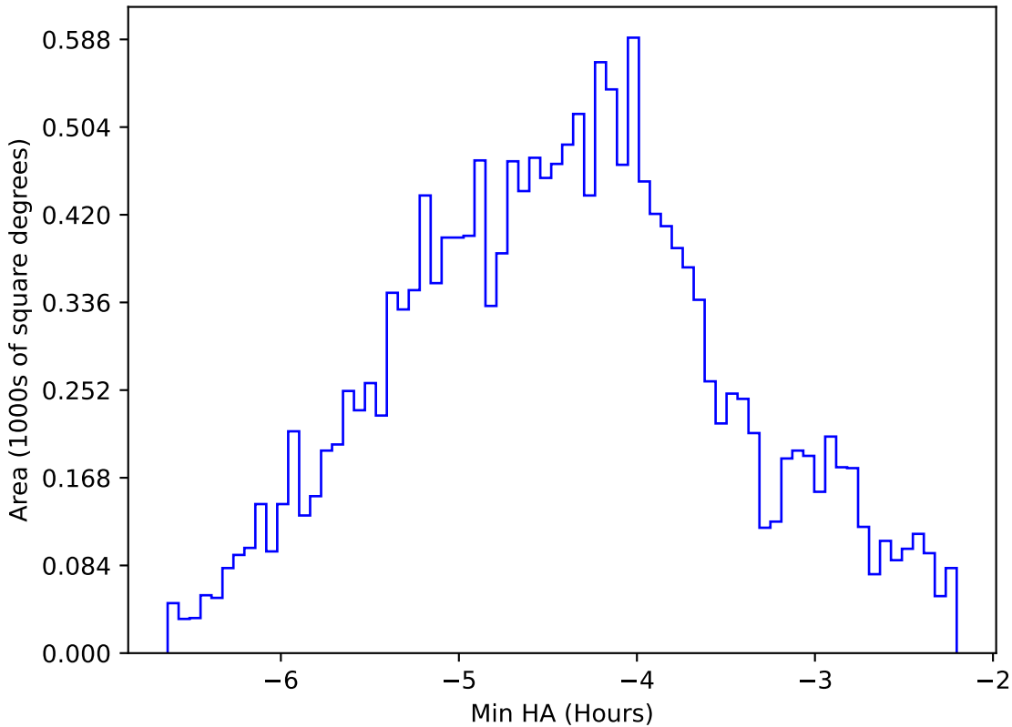
weather_cloudso2v3.4_10yrs WFD i band: Min HA
