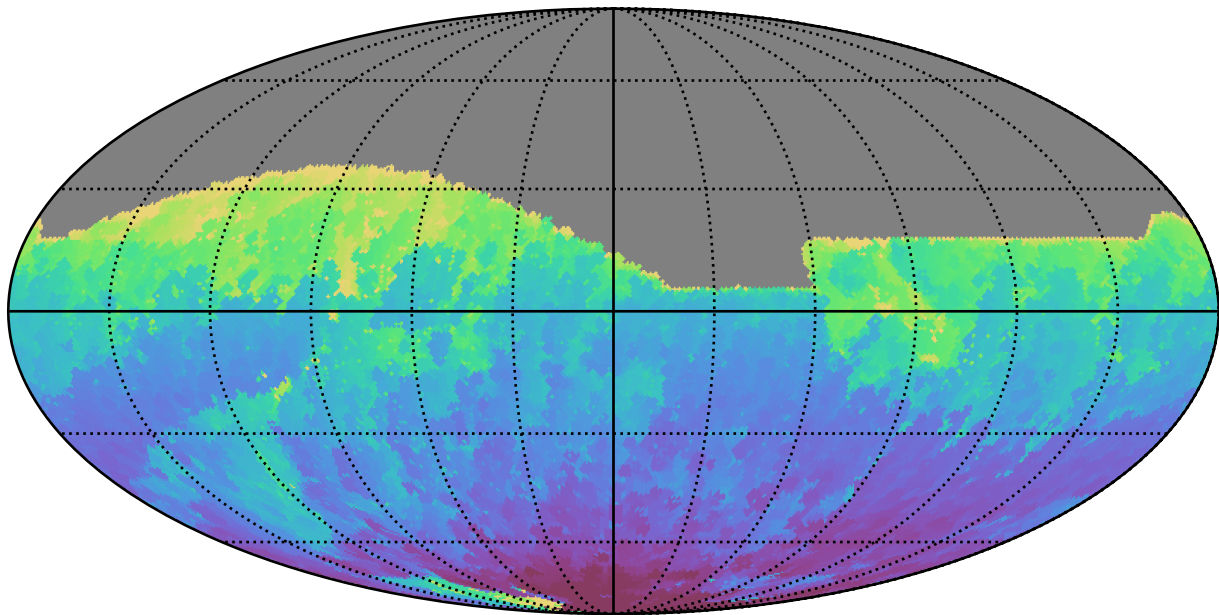
weather_cloudso2v3.4_10yrs All sky z band: Min HA
