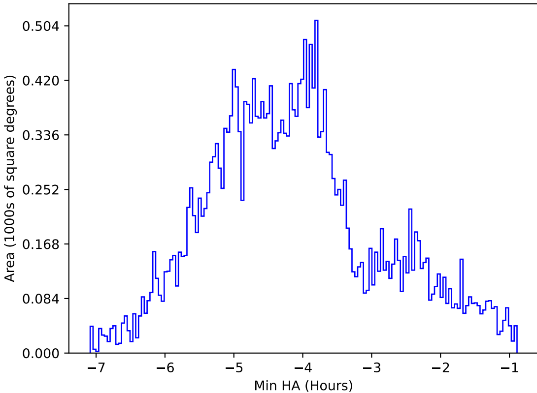
weather_cloudso2v3.4_10yrs All sky z band: Min HA
