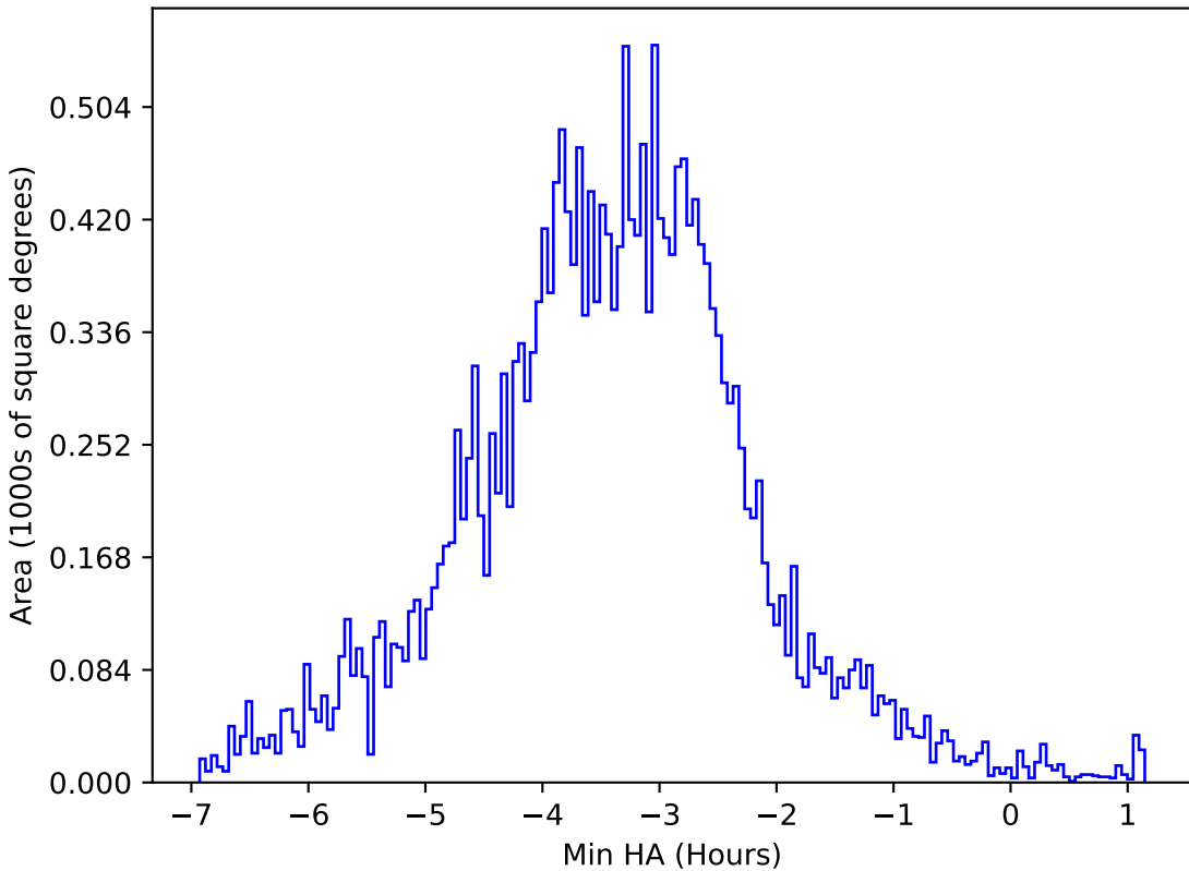
weather_cloudso2v3.4_10yrs All sky y band: Min HA
