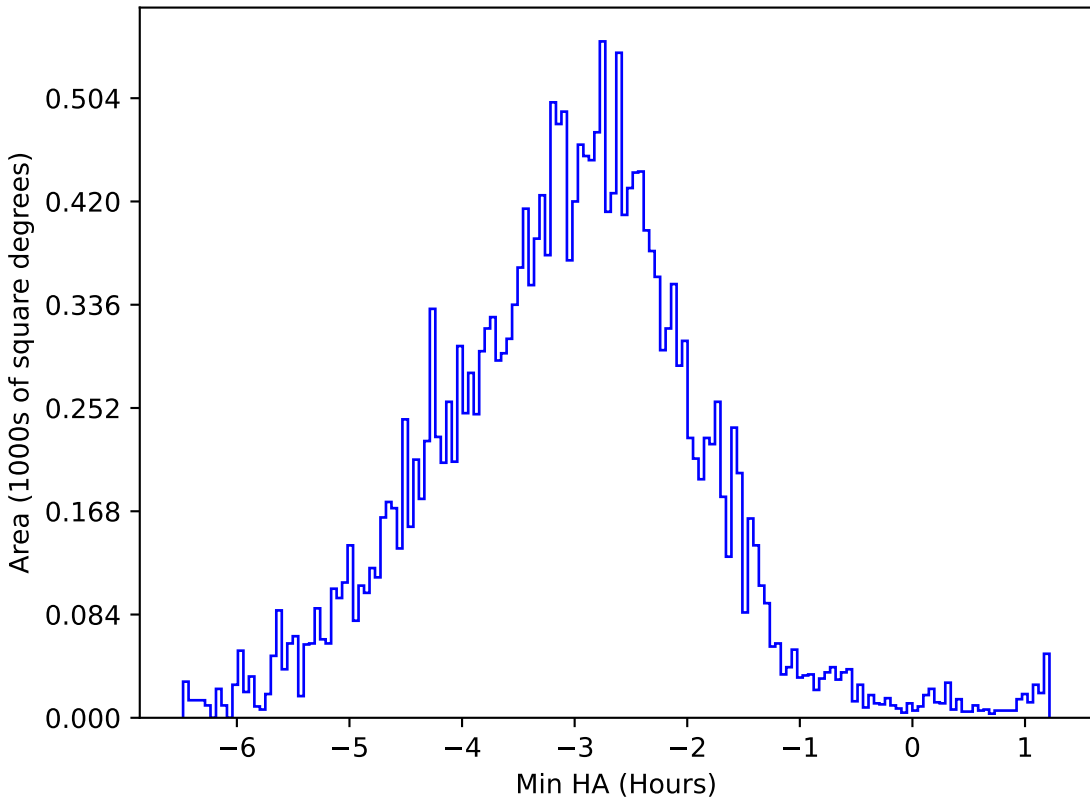
weather_cloudso2v3.4_10yrs All sky u band: Min HA
