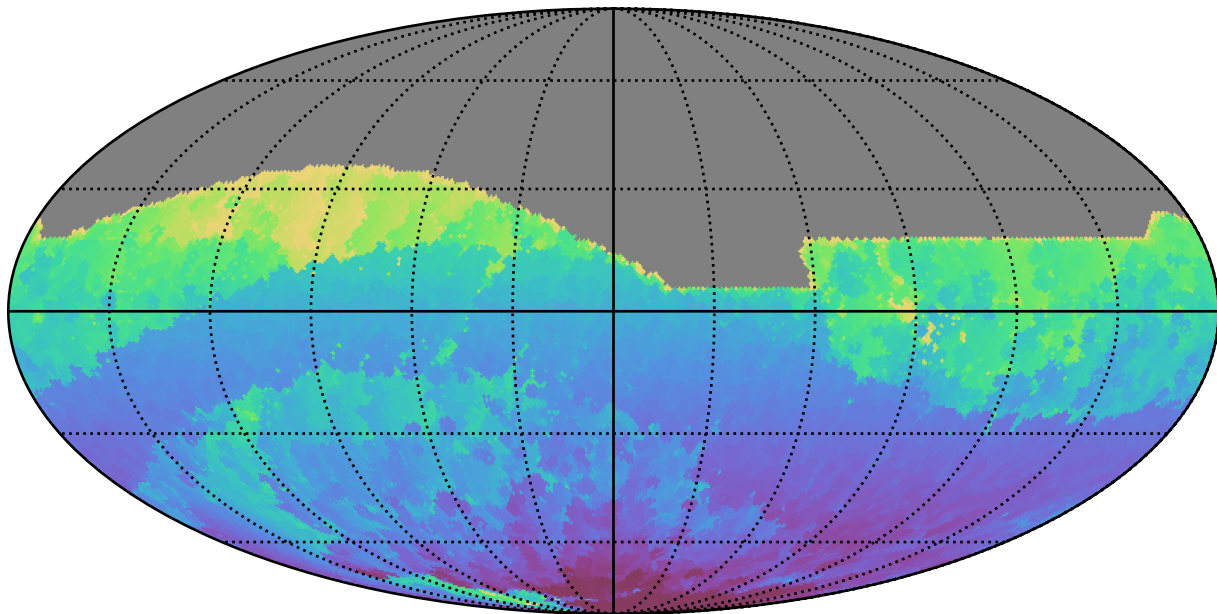
weather_cloudso2v3.4_10yrs All sky r band: Min HA
