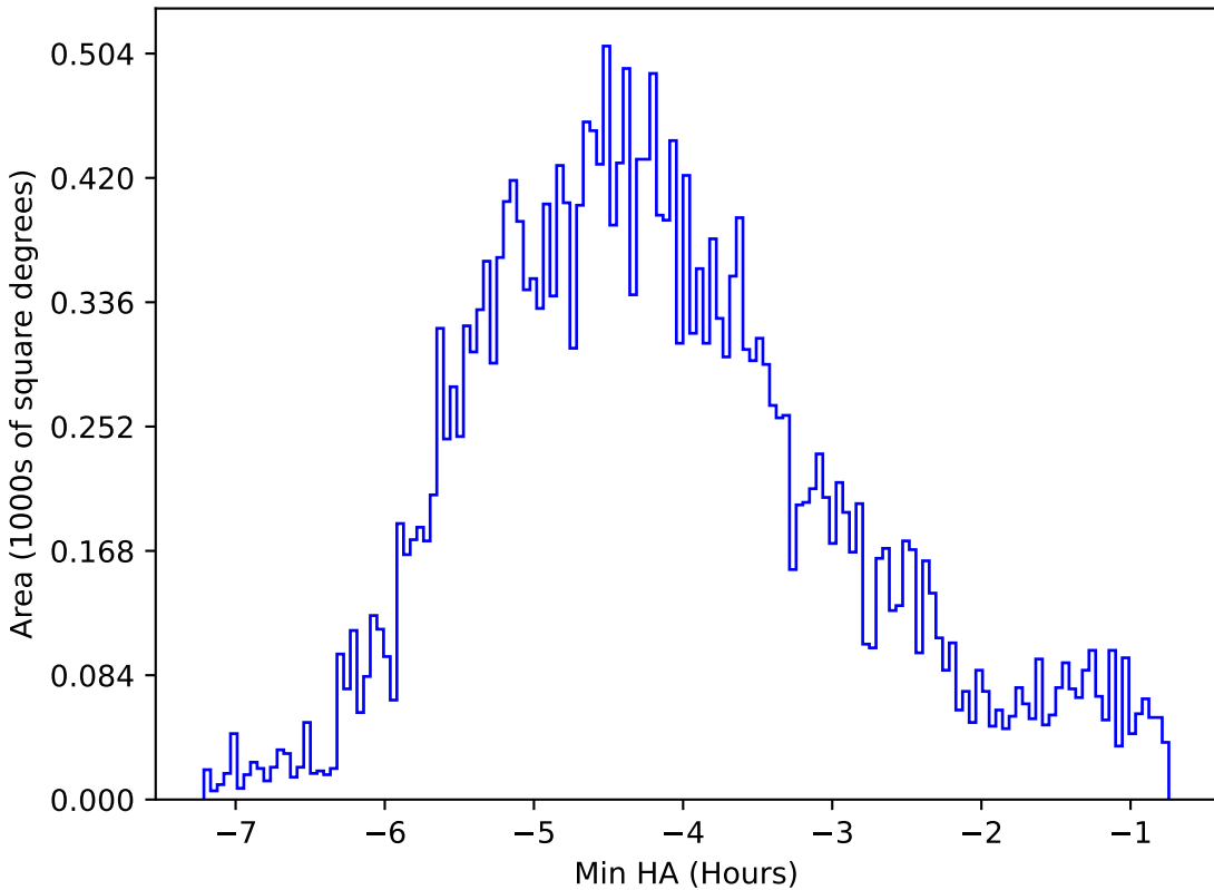
weather_cloudso2v3.4_10yrs All sky r band: Min HA
