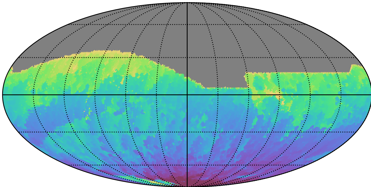
weather_cloudso2v3.4_10yrs All sky i band: Min HA
