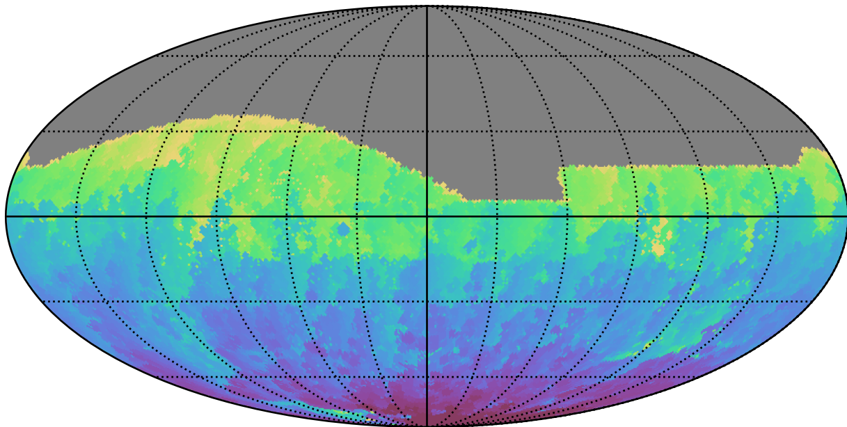
weather_cloudso2v3.4_10yrs All sky g band: Min HA
